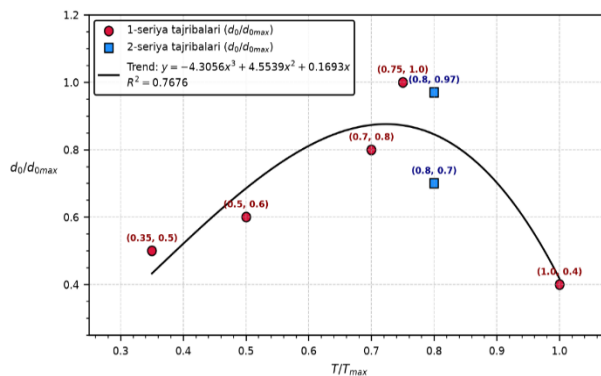
5-rasm. Bog'langan grunt agregati uzilishini vaqtga bog'liq ravishda
