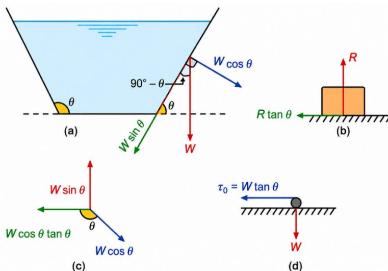
2-rasm. Kanal qiyaliklarida ta'sir etuvchi kuchlar.
