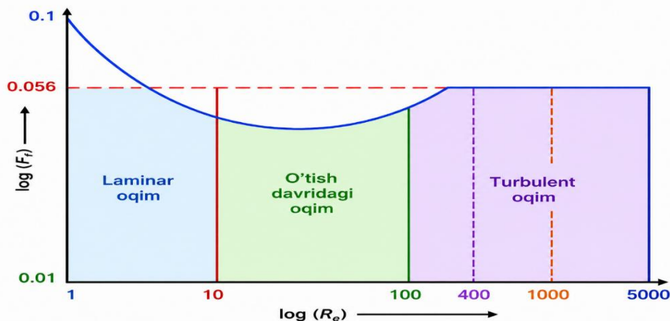
6-rasm. F_s va R_c orasidagi bog'liqlik
