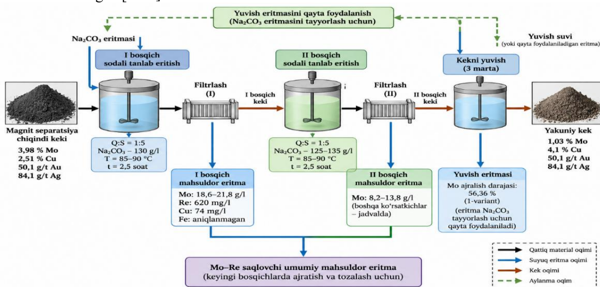
2-rasm. Magnit separatsiya chiqindilarini ikki bosqichli sodali tanlab eritishning tavsiya etilayotgan texnologik sxemasi.
