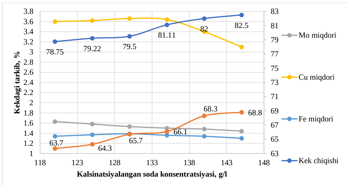
1-rasm. \text{Na}_2\text{CO}_3 konsentratsiyasining molibdenning eritmaga ajralish darajasiga ta'siri.
